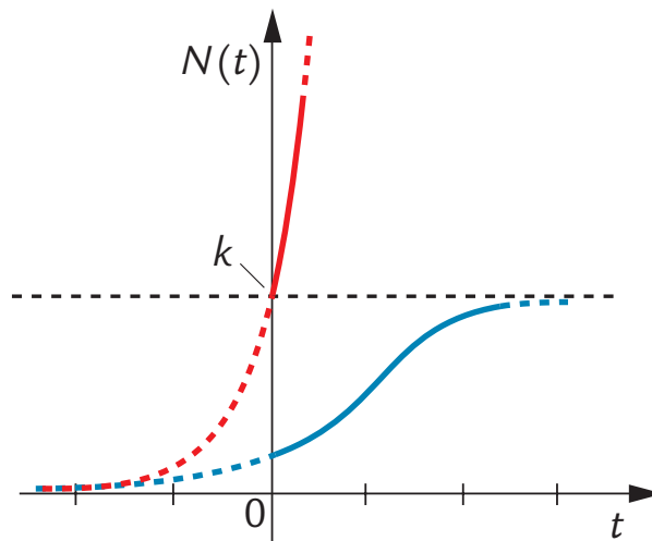
Figura 2 Confronto fra la curva logistica e la curva di accrescimento esponenziale.
