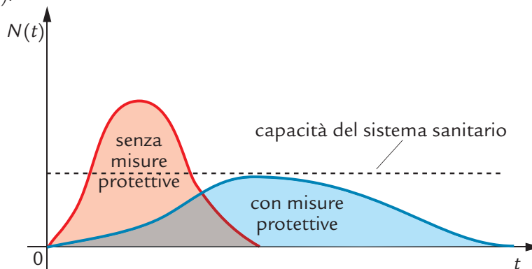
Figura 3 Il grafico “abbatti la curva”, diventato virale durante l'epidemia da nuovo coronavirus.
